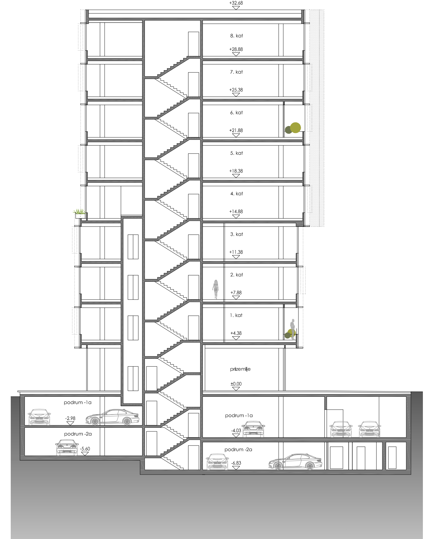
PRESJEK 2 1:200
